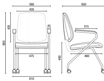
43.106 Z ROD Executiva Aproximação
